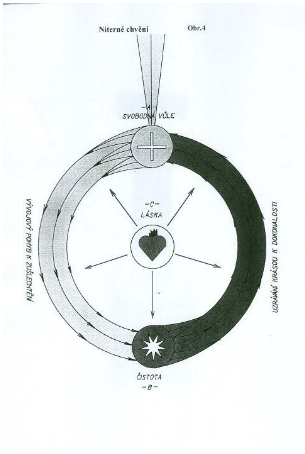
Obrázek 4. Niterné chvění
